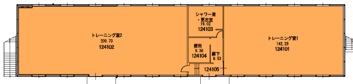
第4クラブハウス1階
