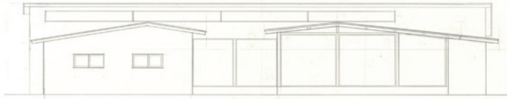
東立面図 1/100
