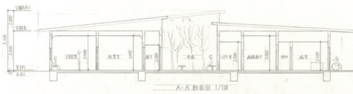
A-A' 断面図 1/100
