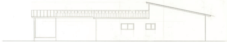
北立面図 1/100
