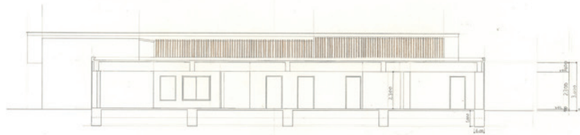
XX側面図 1/100
