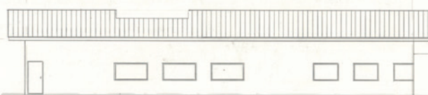
西立面図 1/100
