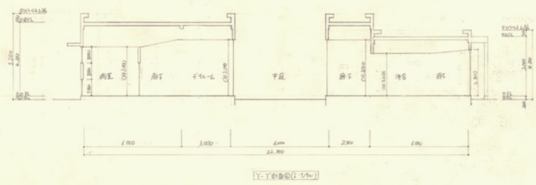
1階平面 (22.80m)
