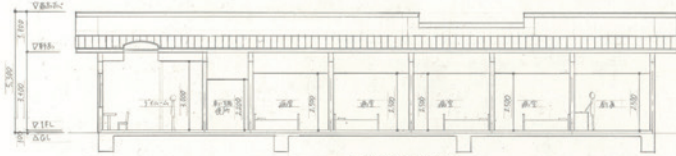
B-B' 断面図 1/100
